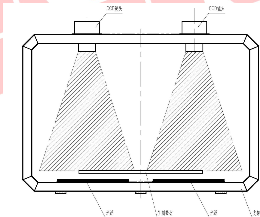
图 1 CPC 检测示意图
